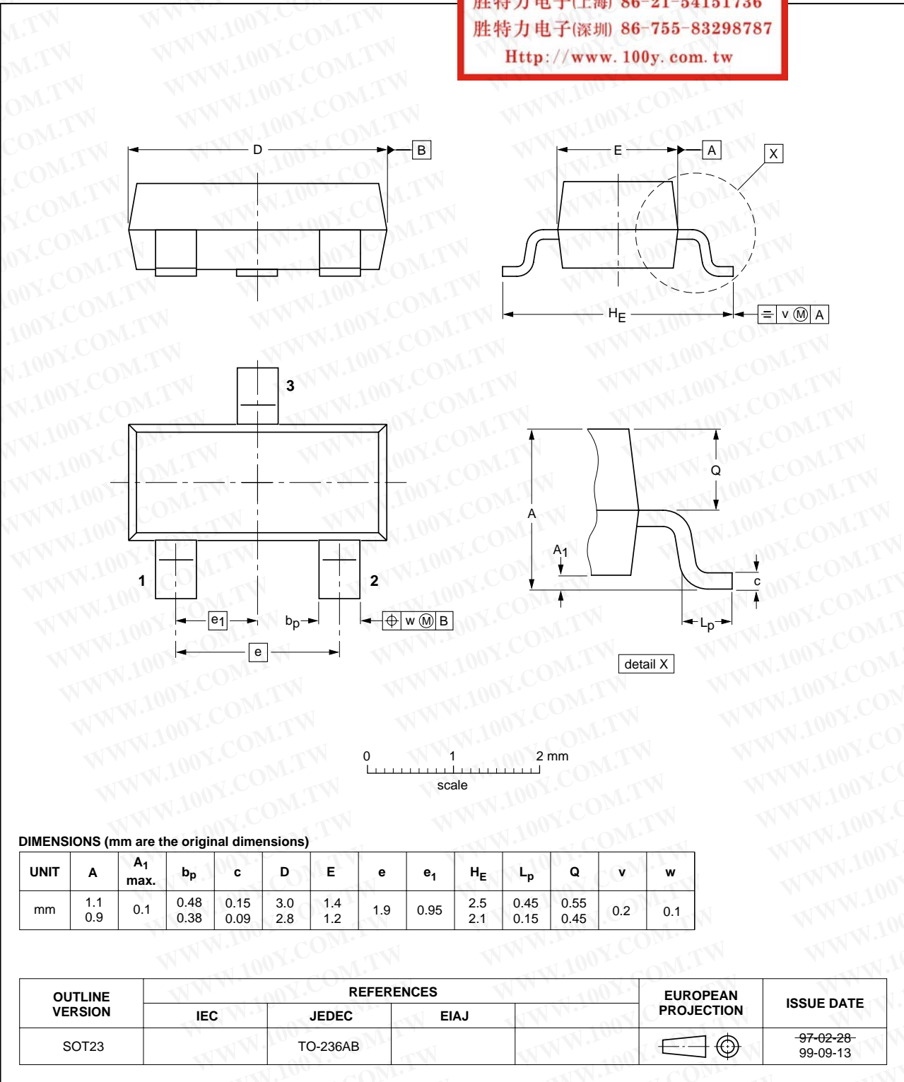
Fig 14. SOT23.
