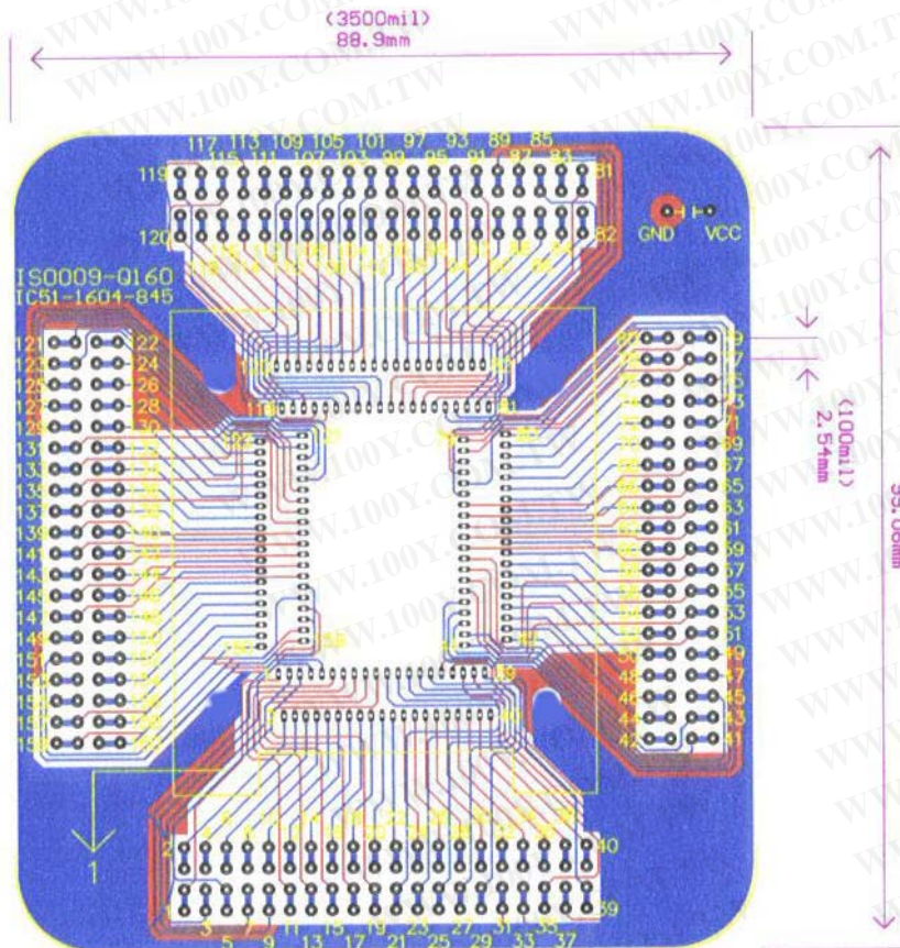
QFP160/DIP160
