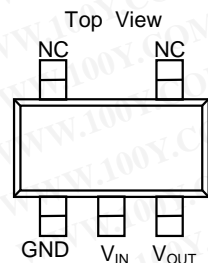
(3) SOT-23-5
