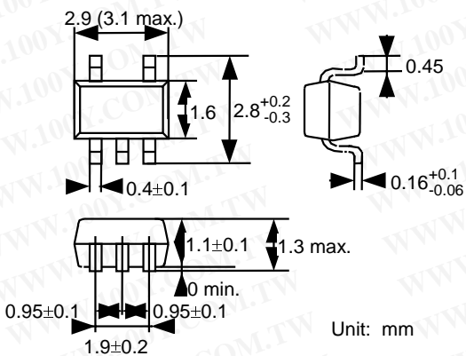
(3) SOT-23-5
