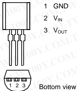
(1) TO-92
