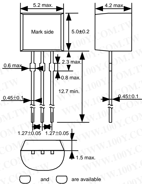
(1) TO-92
