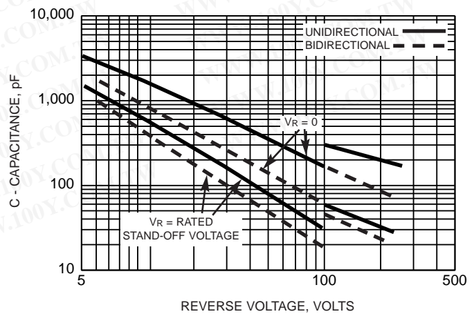
FIG. 6 - CAPACITANCE
