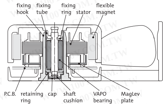
MagLev AC Fan Structure
