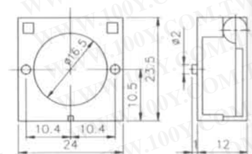
● 固定圈鎖緊與燈泡裝卸器 T16-A
