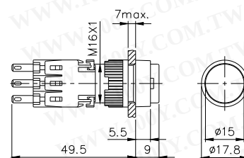
TN16-ABR/MBR
