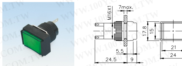
TN16-PIL/PLL/PNL
