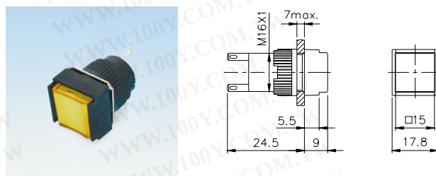
TN16-PIL/PLL/PNL
