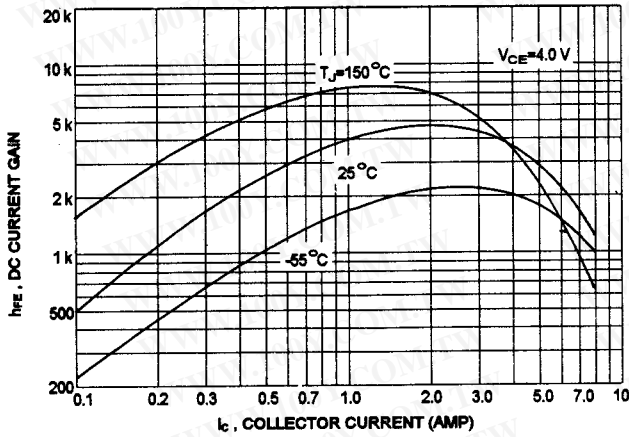
NPN TIP120,TIP121,TIP122
