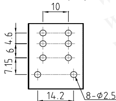
SPDT (1C)
