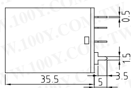
P.C.B Terminal Type
