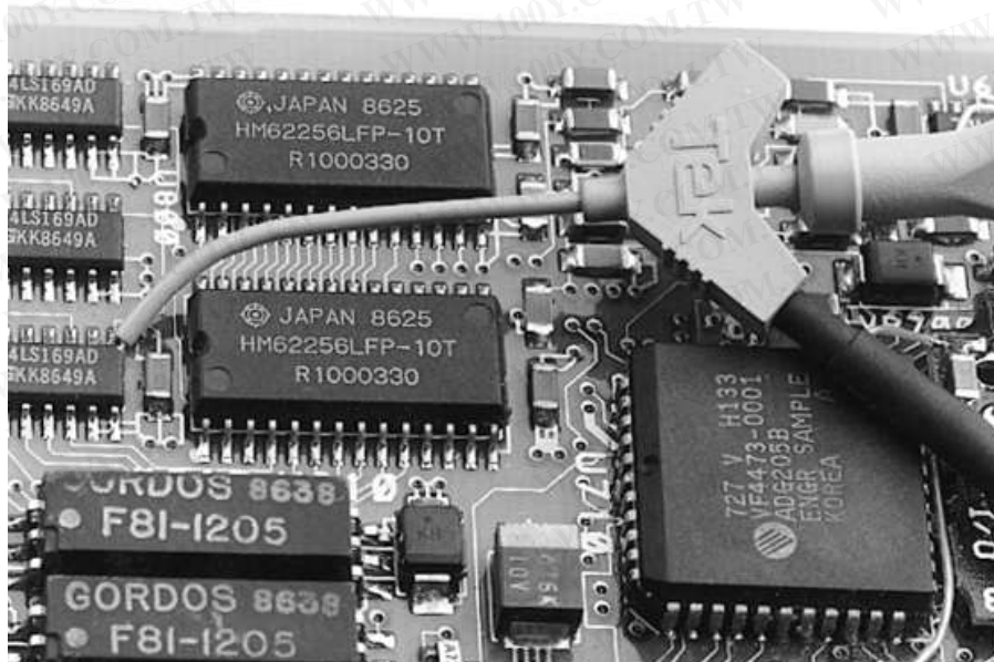
SMT KlipChip Adapter.
