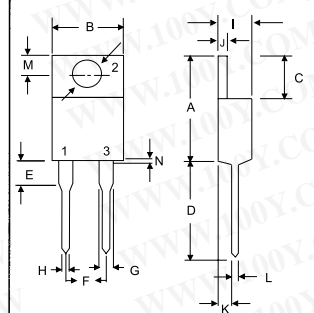
TO-220A
