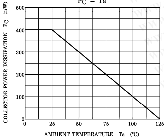
P_C - T_a
