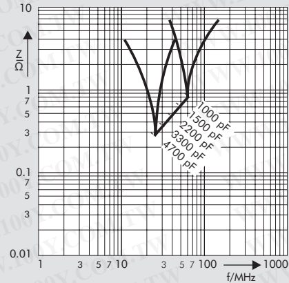
Scheinwiderstand in Abhängigkeit von der Frequenz (Richtwertel). Impedance change with frequency (general guide).
