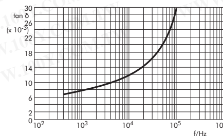
Verlustfaktor in Abhängigkeit von der Frequenz (Richtwertel) Dissipation factor change with frequency (general guide)
