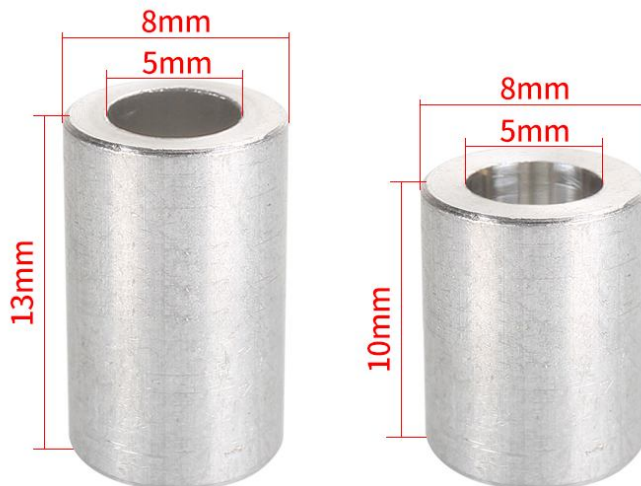
滑轮隔离柱尺寸
