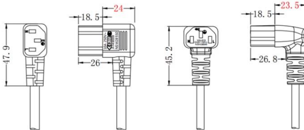
IEC320 C13 左/右弯尺寸图
