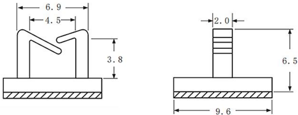
测量示意图
