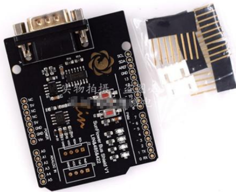
HW-A2 Arduino扩展Lin 485 422总线 模块
