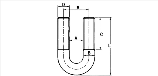
测量示意图
