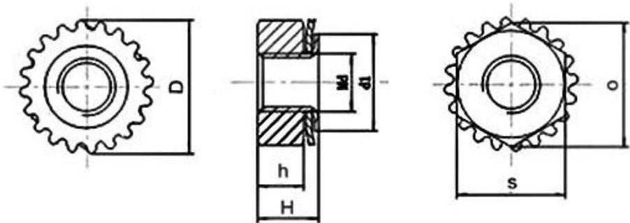
測量示意图
