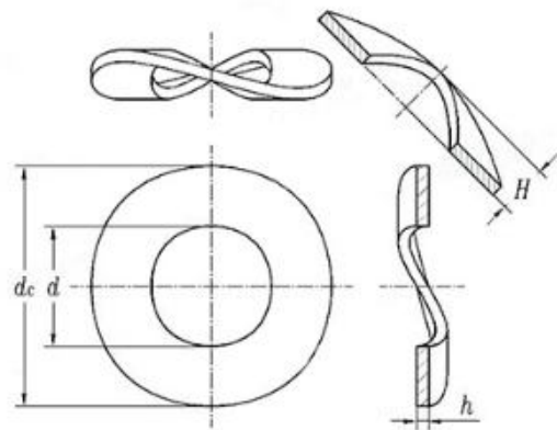
測量示意图
