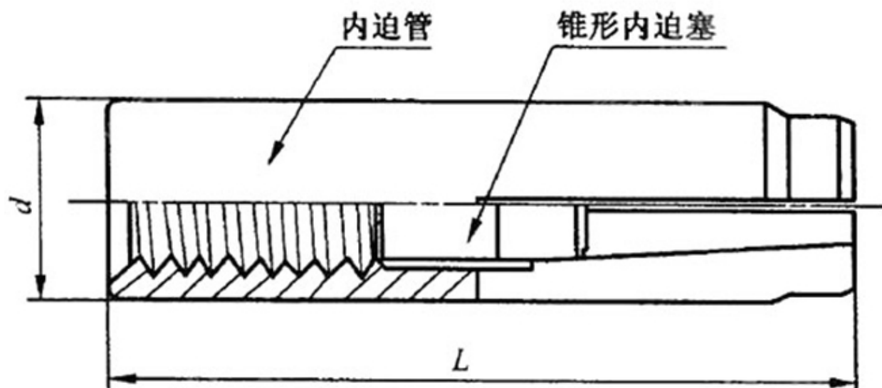
測量示意图
