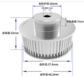
60齿内孔5mm(带宽10mm)
