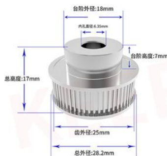
40齿内孔6.35mm(带宽6mm)
