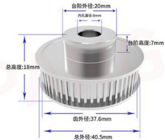
60齿内孔8mm(带宽6mm)
