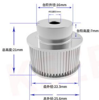
36齿内孔5mm(带宽10mm)
