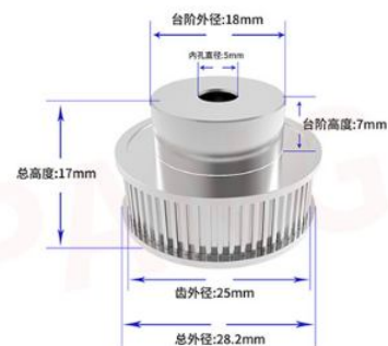
40齿内孔5mm(带宽6mm)
