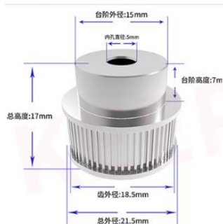
30齿内孔5mm(带宽6mm)
