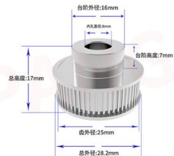
40齿内孔8mm(带宽6mm)
