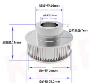
40齿内孔10mm(带宽6mm)
