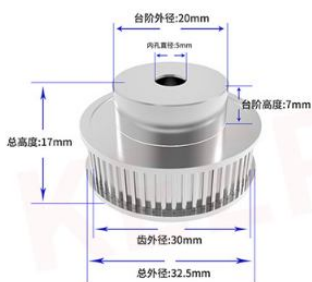
48齿内孔5mm(带宽6mm)
