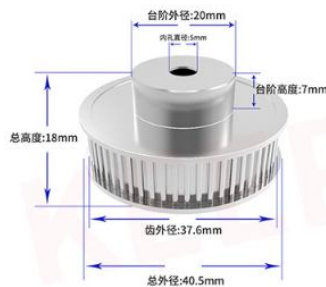
60齿内孔5mm(带宽6mm)
